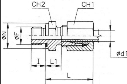
FORMA E DIN 3852
